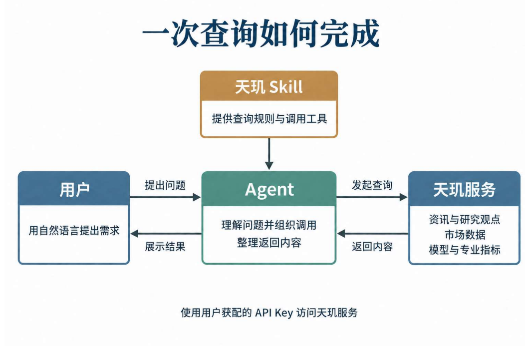
图 4 天玑服务的调用过程
